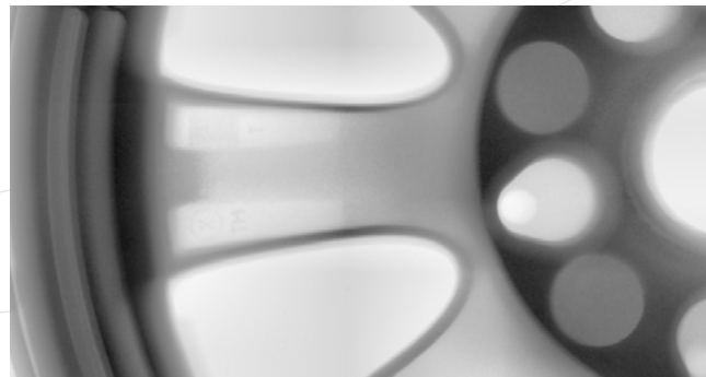
Röntgenbild eines Rades, aufgenommen mit dem Detektor XEye vom Fraunhofer IIS.
